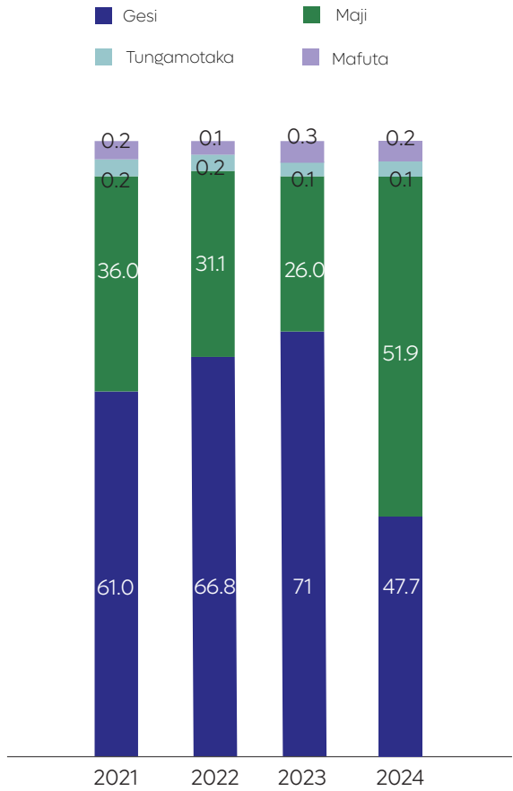
Kielelezo Na. 9.3: Mwenendo wa Mchango wa Umeme uliozalishwa katika Gridi ya Taifa kutoka Vyanzo Mbalimbali, Mwaka 2021-2024
